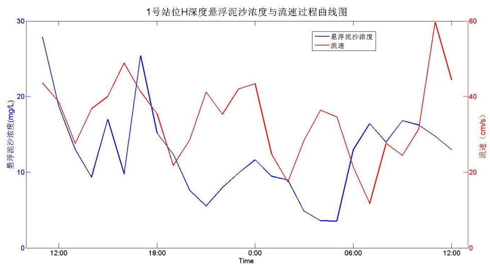
图 5.6-25 1 号站 H 深度悬浮泥沙浓度与流速过程曲线图
