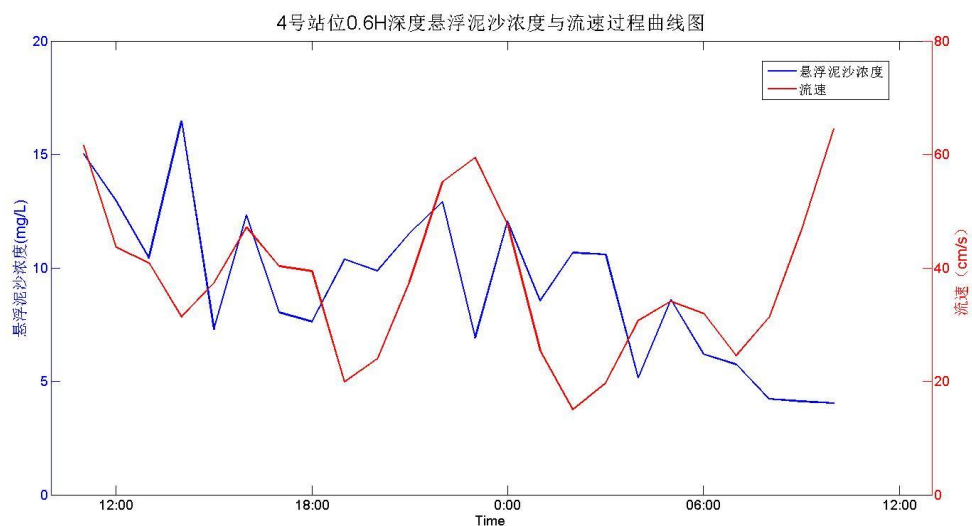
图 5.6-27 4 号站 0.6H 深度悬浮泥沙浓度与流速过程曲线图
