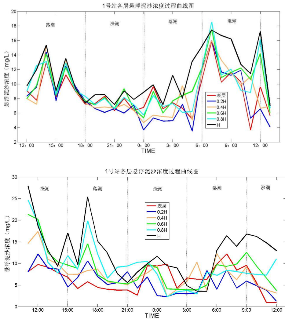
图 5.6-29 两次调查 1 号站各层深度悬浮泥沙浓度过程曲线图 (H 表示水深, 上图 of 第一次调查, 下图为第二次调查)
