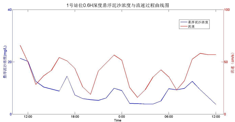
图 5.6-24 1 号站 0.6H 深度悬浮泥沙浓度与流速过程曲线图
