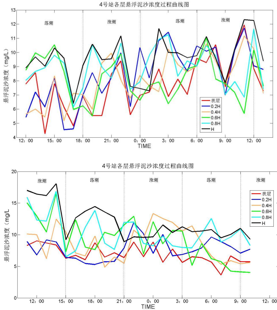
图 5.6-30 4 号站各层深度悬浮泥沙浓度过程曲线图
