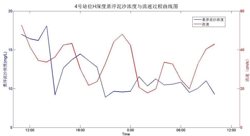
图 5.6-28 4 号站 H 深度悬浮泥沙浓度与流速过程曲线图
